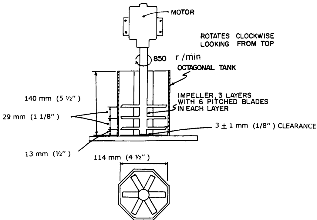
FIG. 1 Attrition Machine
